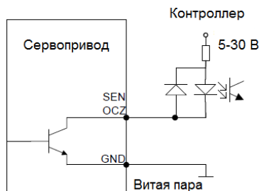
Пример цепи с оптопарой
