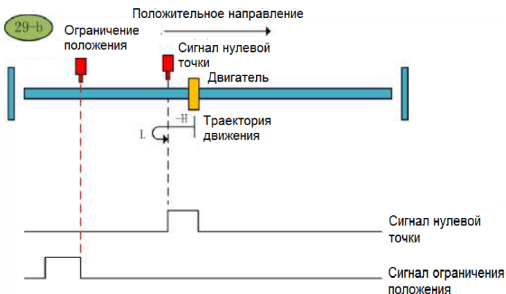
Метод возврата в нулевую точку 29-б
