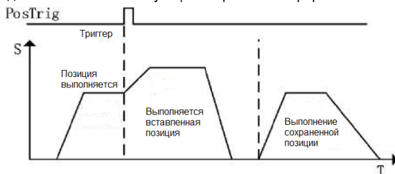
Диаграмма сохранения с прерыванием
