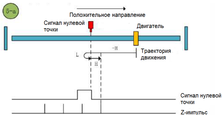
Метод возврата в нулевую точку 5-а
