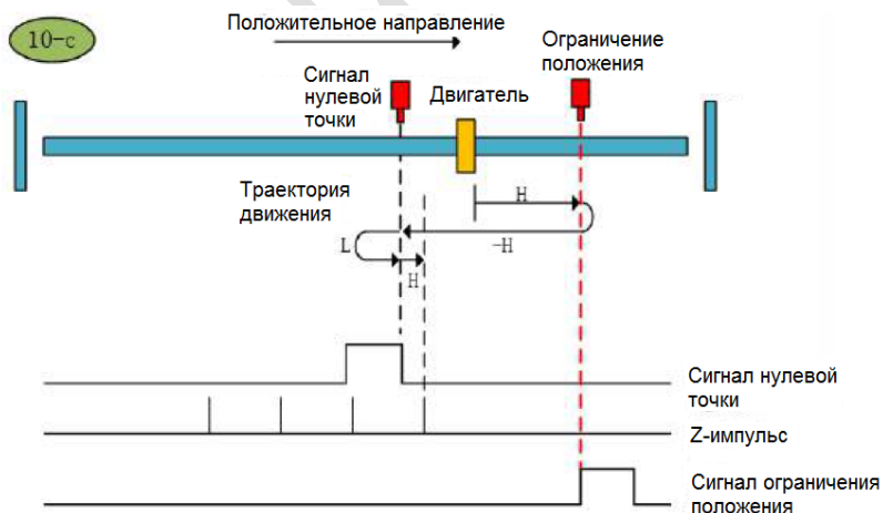
Метод возврата в нулевую точку 10-c
