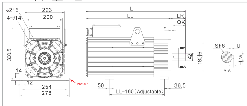
Фланец 200 (Ед.: мм):
