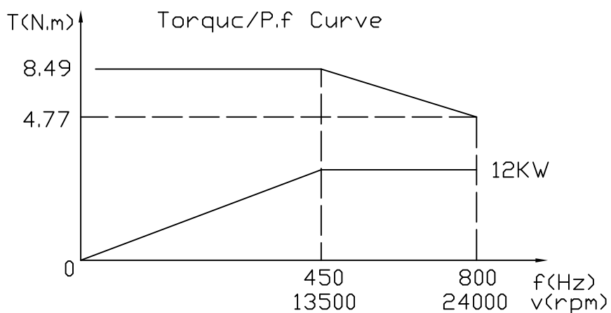
扭矩/功率曲线 Torque/P.f Curve
