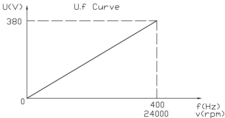
频压曲线
